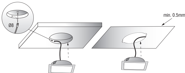
(A) Installazione su legno Fitting - Wooden Surfaces Montage - Holz
