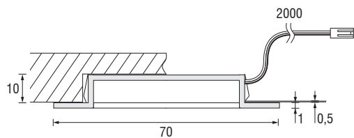
(A) Installazione su legno Fitting - Wooden Surfaces Montage - Holz
