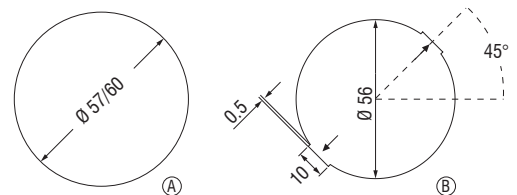
Foro di incasso / Recessed hole / Einbaumaße
